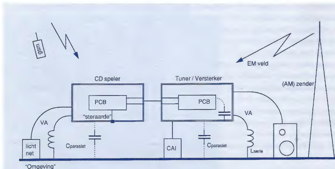
Figuur 4 Aangesloten kabels op een systeem, mogelijke paden voor CM stromen
